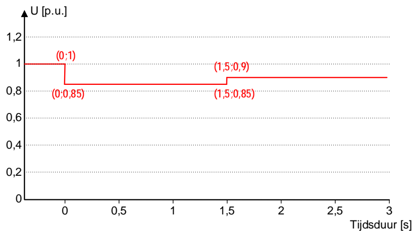
Figuur 13 – Spanning-tijd-profiel voor een noodvoedingssysteem
