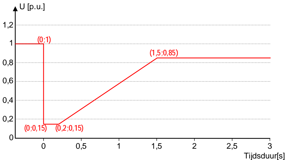
Figuur 12 - Spanning-tijd-profiel voor niet-synchrone productietechnologie (power park module)
