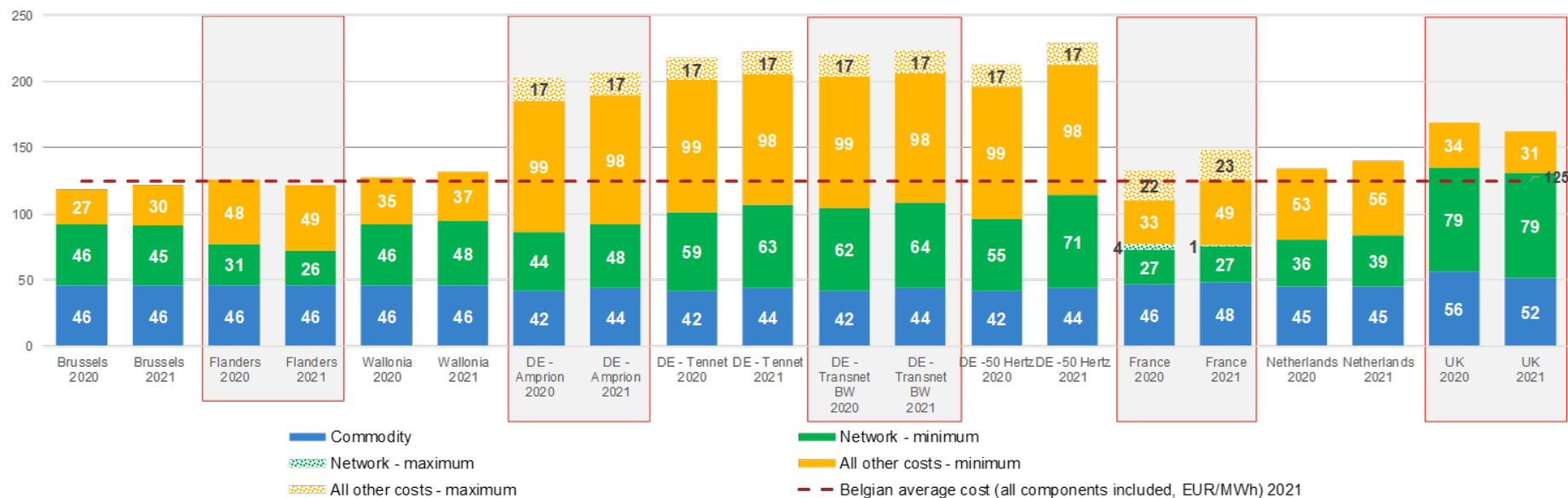
Coût de l'électricité par composante en EUR/MWh (profil E-BSME)
