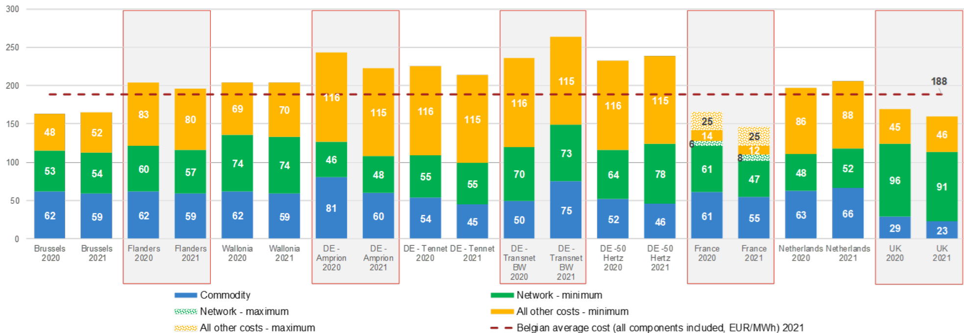
Elektriciteitsprijzen per component in EUR/MWh (profiel E-SSME)
