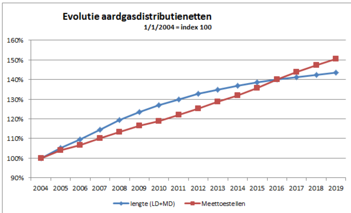
Figuur 10 Evolutie groei aardgasdistributienet en aansluitingen
