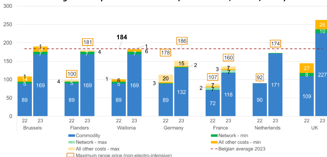
Figuur 3. Elektriciteitsfactuur voor een industrieel bedrijf met een verbruik van 500 GWh/jaar, aangesloten op het transmissienet (2022 en 2023, in euro/MWh)
